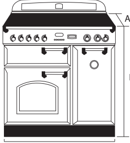
90cm Dual Fuel A: 608 / 670mm B: 905 - 930mm C: 900mm C A: Depth Ex / Inc Handles
